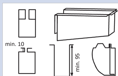
Przykłady gięcia HSBM z wysokim licem górnym, szyną segmentową lub stopką
