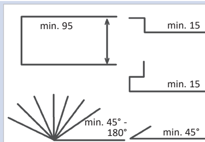
Przykłady gięcia: HSBM z niskim i wysokim licem górnym
