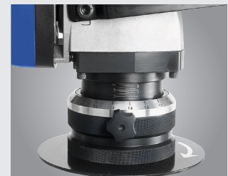
Bezstopniowo ustawiania szerokość fazki 0 - 10,6 mm wygodne i precyzyjne ustawianie szerokości fazki dzięki czytelnej skali 3 kąty fazki 30° / 37,5° / 45°
