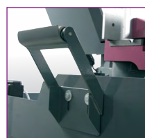
Podpora rolkowa · Do podparcia długich materiałów
