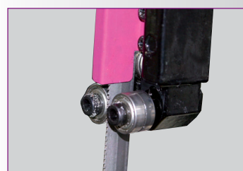
Prowadnica taśmy piły • 3-punktowa prowadnica na łożyskach kulkowych daje znakomite prowadzenie taśmy i tym samym optymalne cięcie
